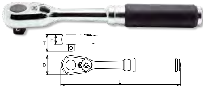
3725Z Reversible Ratchet 3725Z-280
