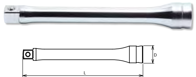
3760Z-75 · -125 · -250 Extension Bars
